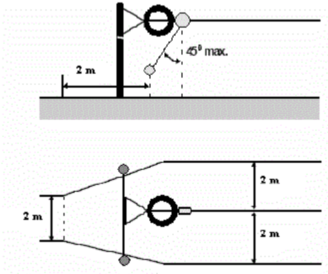
Фиг. 4. Минимална широчина и дължина на ударопогълщаща настилка за въжени линии
